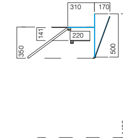
OPÇÃO: VDAP vidro direito alto c/ prateleira e pala higiénica high flat glass w/ shelf and sneeze guard vitrage droit haut avec étagère et para haleine vidrio reto alto c/ estante y anti-estornudos
