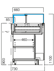
VMINSPOS - VDB UV padaria bakery boulangerie panadería
