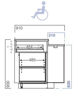
VMINPD P - VDB UV padaria bakery boulangerie panadería
