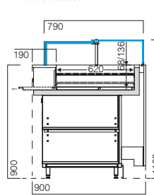
VMINPD B - VDB UV padaria bakery boulangerie panadería
