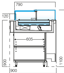
VMINVS - VDB UV 3M2 ventilada superior upper ventilated ventilée supérieure ventilada superior
