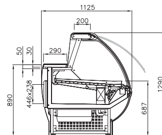
PTRV - VCV-CH ventilada com tampo refrigerado fan assisted w/ piped deck ventilée avec froid contact ventilada con tampo refrigerado
