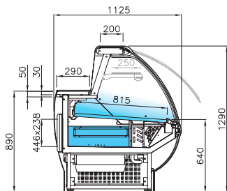
PRC - VCV-CH 3M1 talho e charcutaria meat and delicatessen viande et charcuterie carne y charcutería
