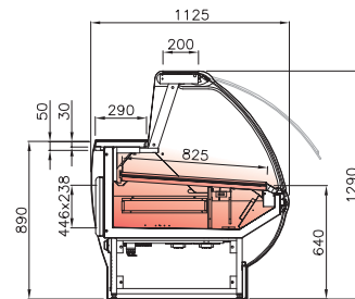
PTAV - VCV-CH ventilada com tampo aquecido fan assisted w/ heated deck ventilée avec plateau chaud ventilada con tampo caliente
