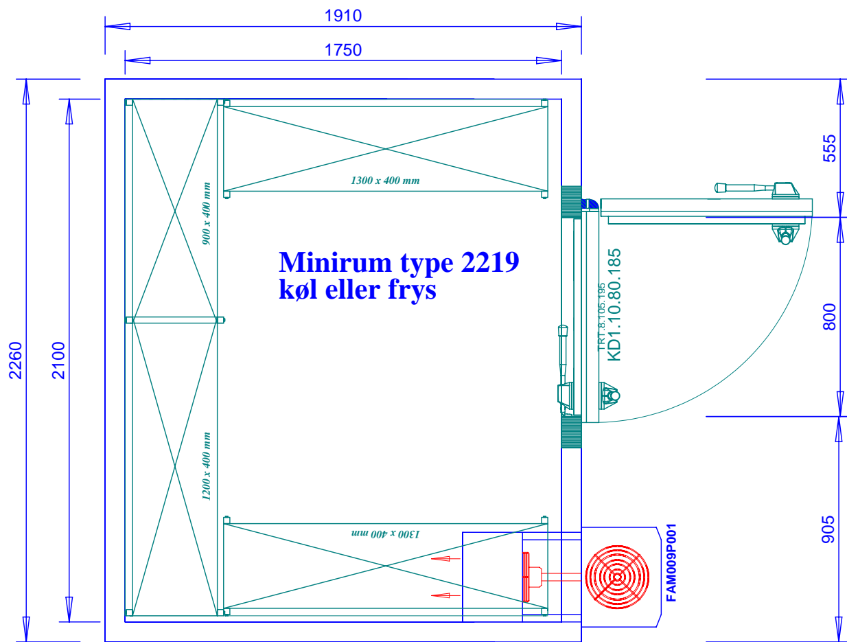
Køleaggregat
