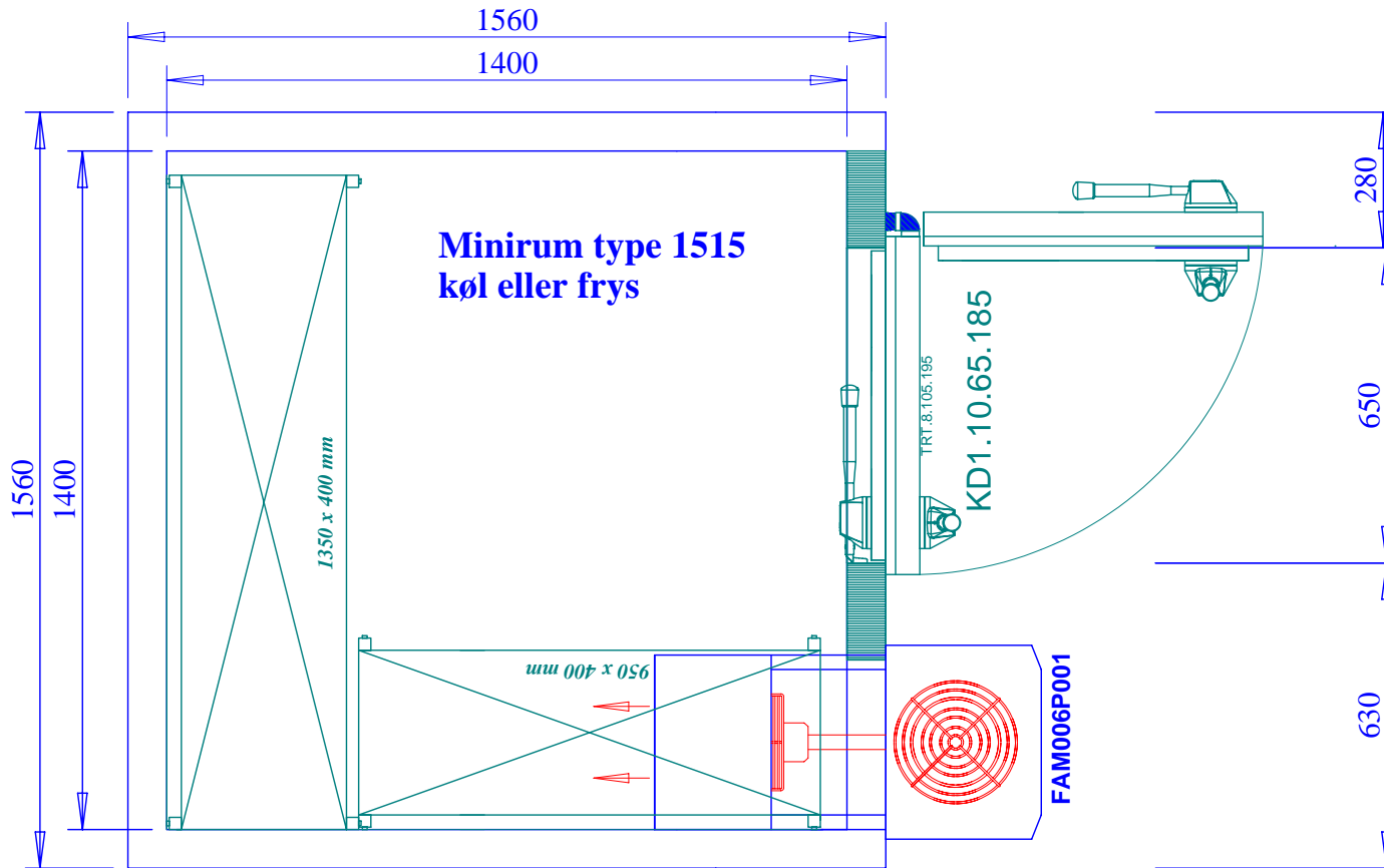
Køleaggregat
