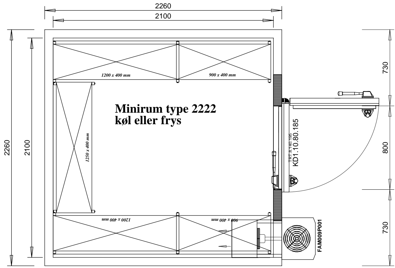
Køleaggregat
