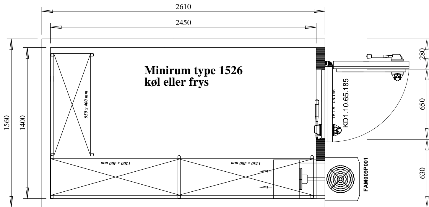
Køleaggregat
